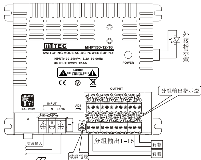
MHP150-12-16 接線示意圖:
