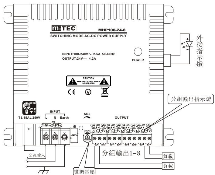
MHP100-24-8 接線示意圖:
