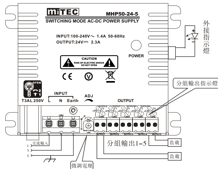
MHP50-24-5 接線示意圖:
