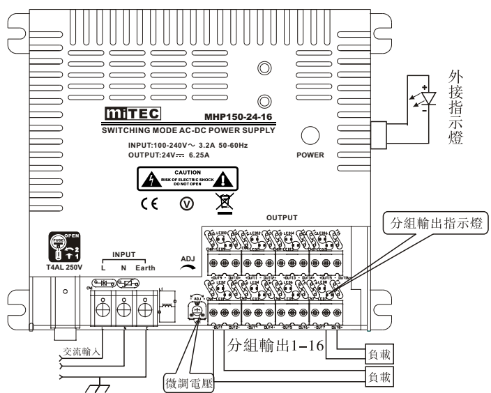
MHP150-24-16 接線示意圖:
